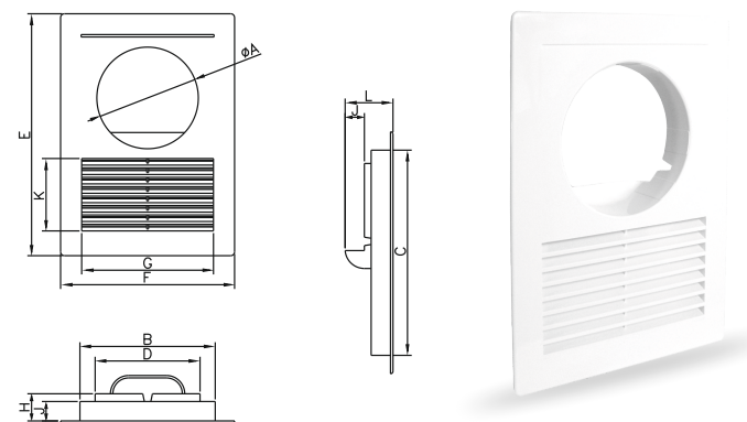
D14/OW KRATKA WENTYLACYJNA - PROSTOKATNA
